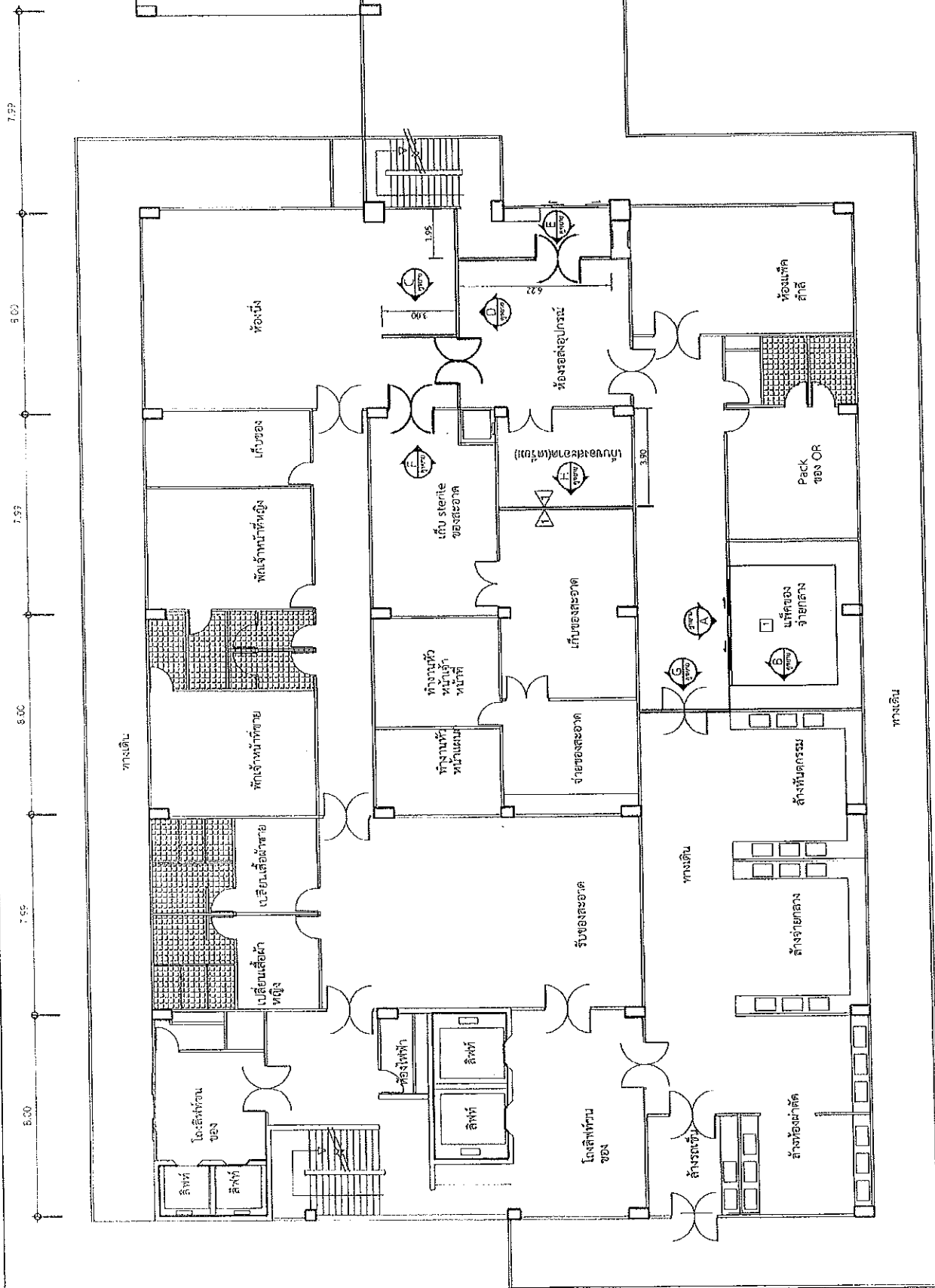
แปลนชั้นที่ 6 หลังปรับปรุง ขนาด 1:250
